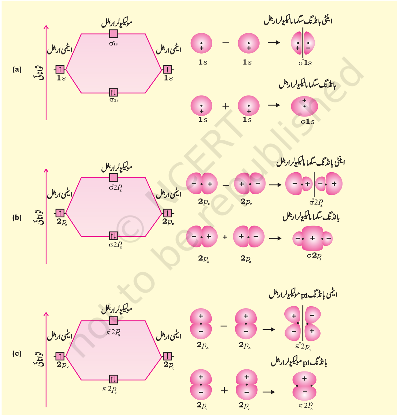
شکل 4.20 (a) 1s ایٹمی اربٹل، (b) 2p_z ایٹمی اربٹل اور (c) 2p_x ایٹمی اربٹل کے اتحاد سے بننے والے بانڈنگ اور اینٹی بانڈنگ مالیکولر اربٹل کی توانائیاں اور خدو خال
