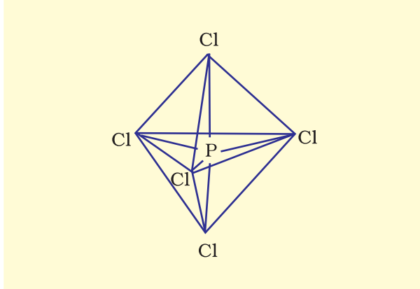
شکل 4.17 \text{PCl}_5 سالمہ کی ٹرائی گونل پیرامیڈل جیومیٹری
