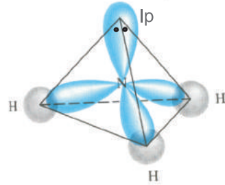
شکل 4.13 NH 3 سالمہ کا بننا
