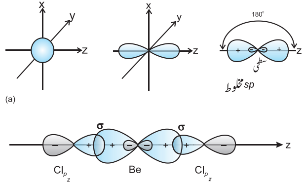
شکل 4.10 (a) s اور p اوریل سے sp مخلوط کا بننا (b) خطی سالمے BeCl_2 کا بننا
