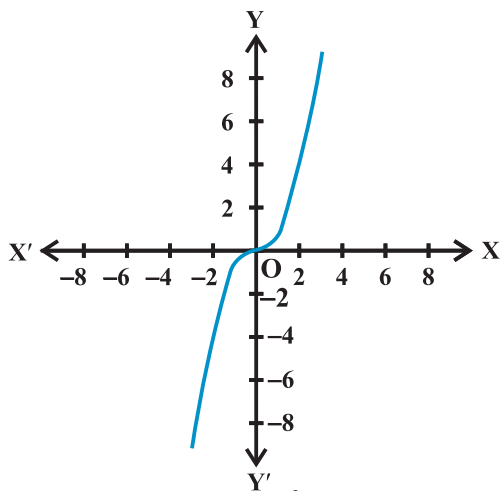
f(x) = x^3 आकृति 2.11
