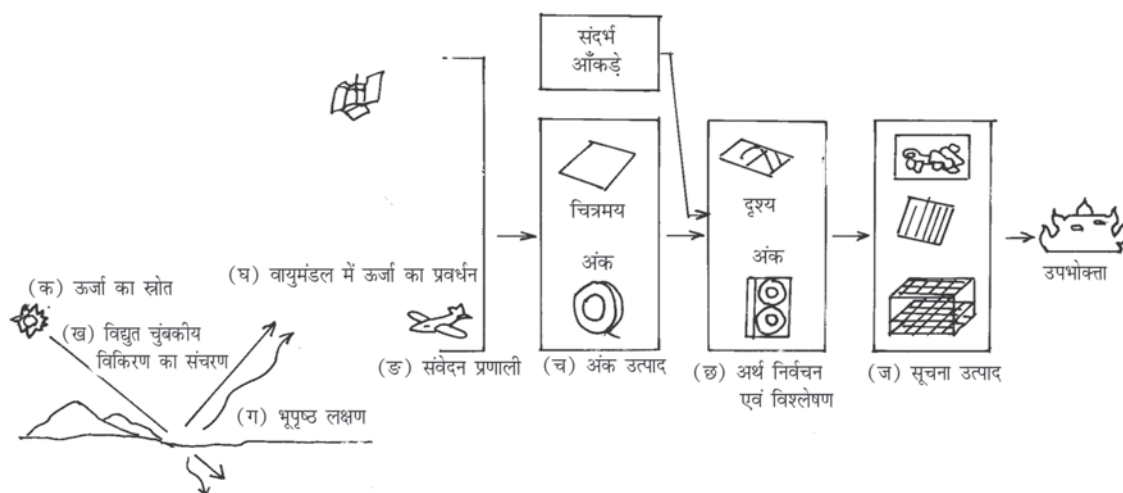
चित्र 7.2 : सुदूर संवेदन के आँकड़े अर्जन करने के चरण
