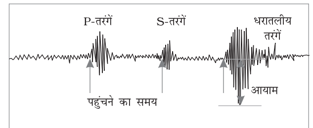
चित्र 3.1 : भूकंप-अभिलेख
