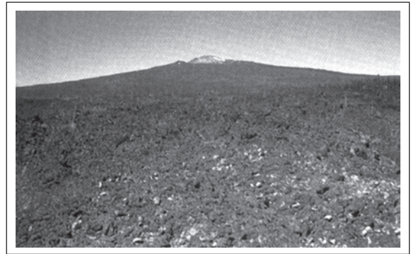
सिंडर शंकु
