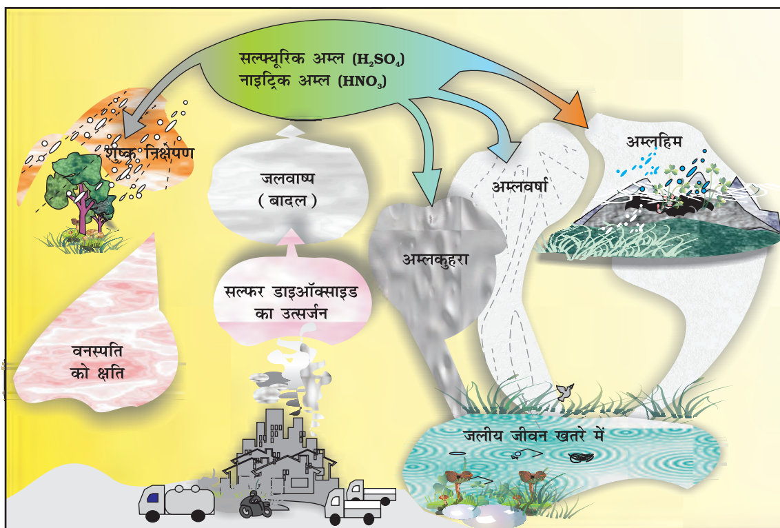
चित्र 14.1 अम्ल-निक्षेपण
